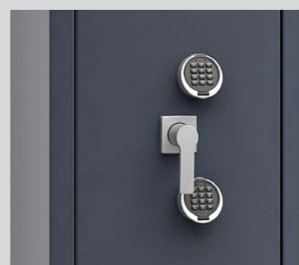
Zamek elektroniczny - Primor 3000 level 5 lub level 15
