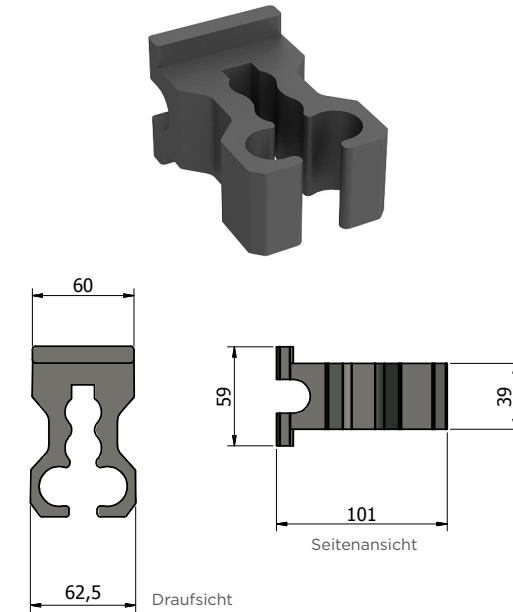
Waffenhalter aus Vollgummi
